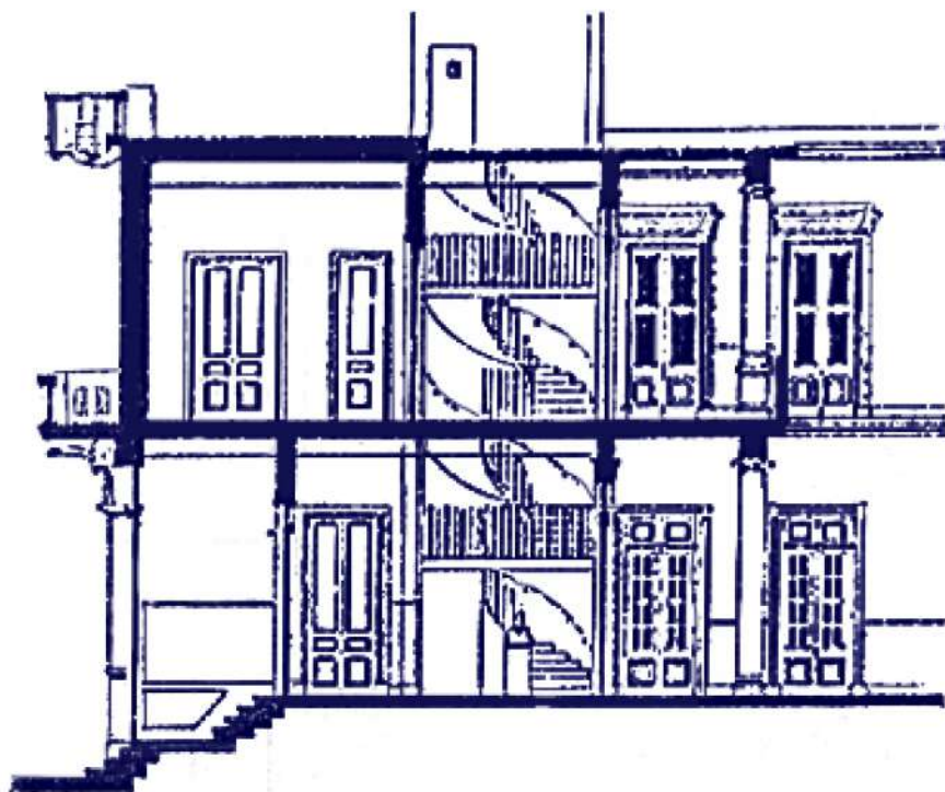
Corte
